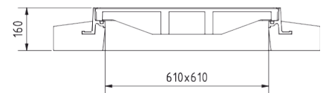
A-A ( 1 : 10 )
